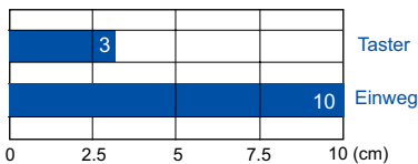
■ Reich-/Tastweite mit Standard Lichtleitern LLK (Kunststoff)
